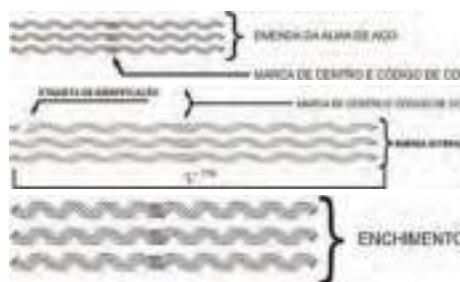
Emenda Preformada Total para Condutores de Alumínio Nu CAA (FULL TENSION SPLICE)
